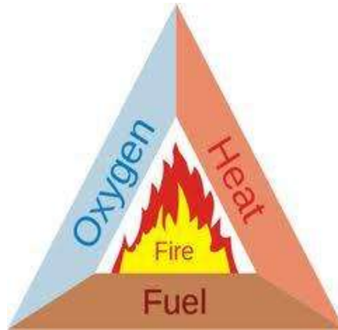
Gambar 1. Segitiga api
